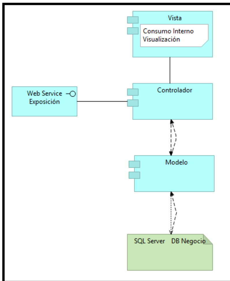
Ilustración 12 Componentes del patrón de arquitectura MVC.
