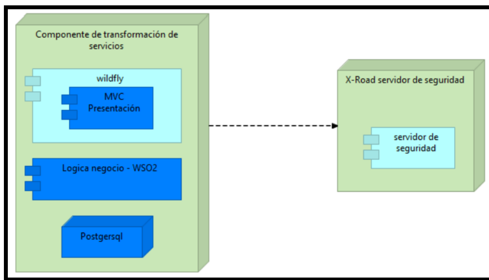
Ilustración 18 Diagrama de despliegue
