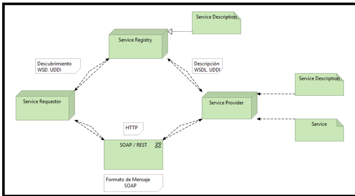
Ilustración 11 Conexiones físicas entre los componentes
