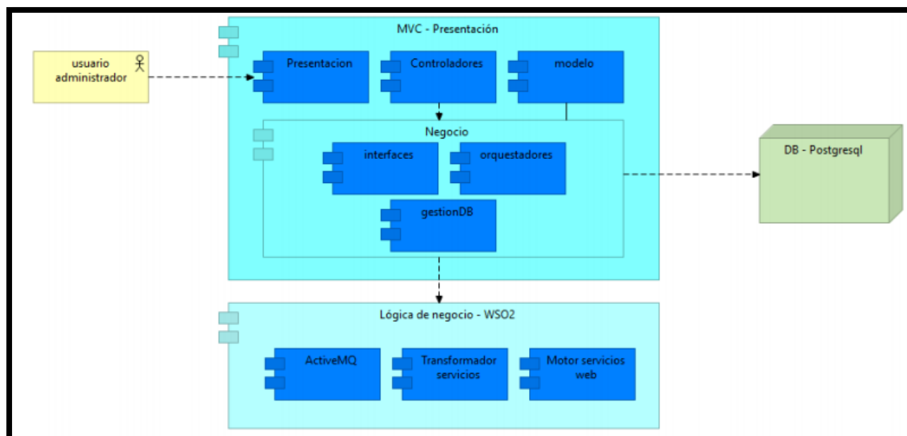
Ilustración 17 Diagrama de componentes
