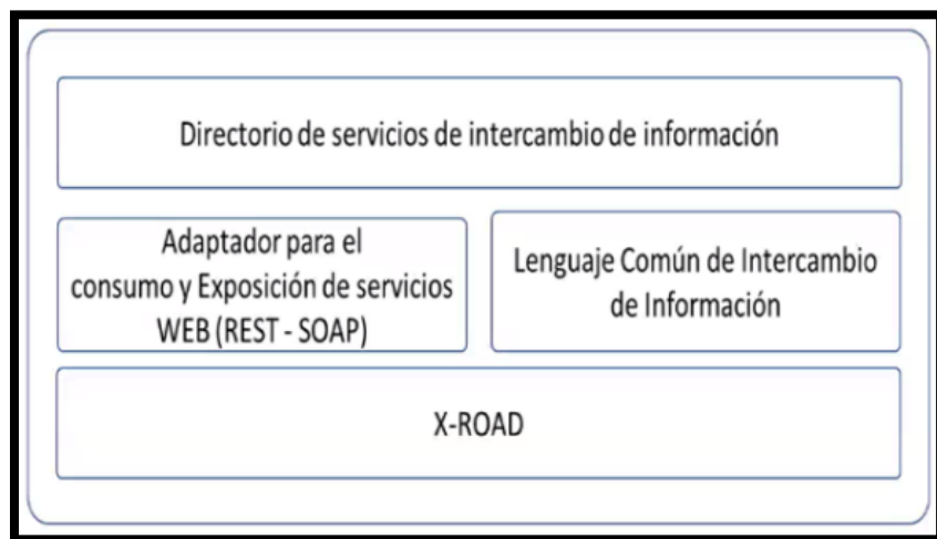
Ilustración 13 Componentes de la Plataforma de Interoperabilidad.
