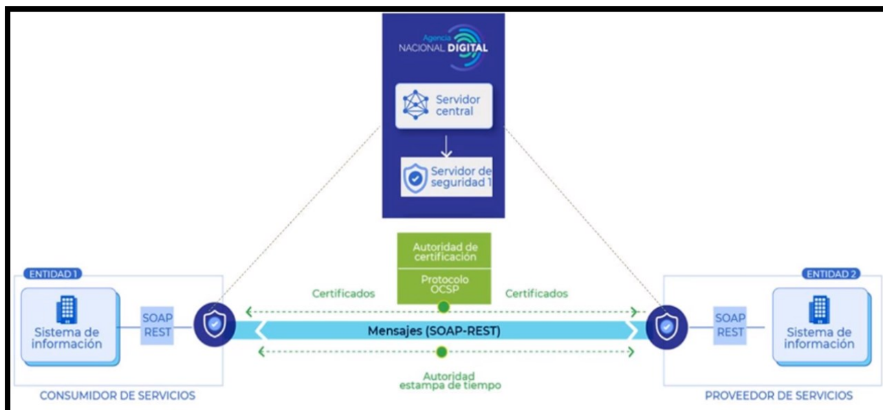
Ilustración 15 Modelo conceptual X-Road
