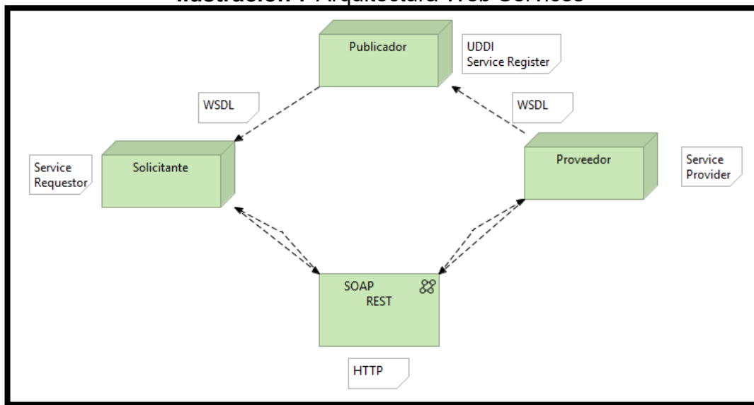
Ilustración 7 Arquitectura Web Services
