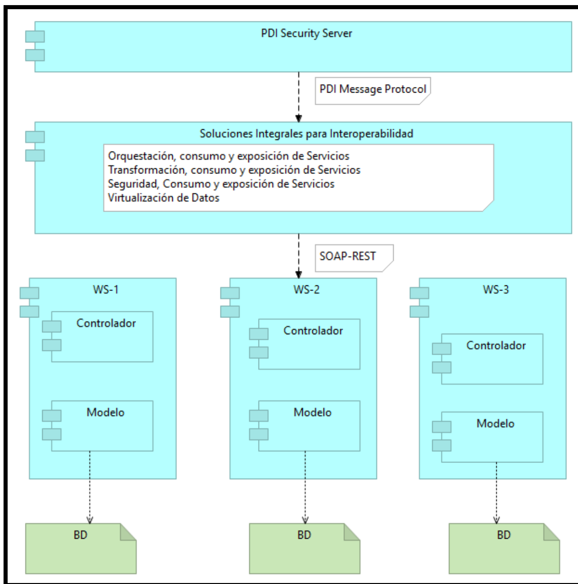
Ilustración 14 Arquitectura implementación de Web Services
