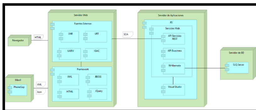
Ilustración 10 Componentes de Software en la capa física.
