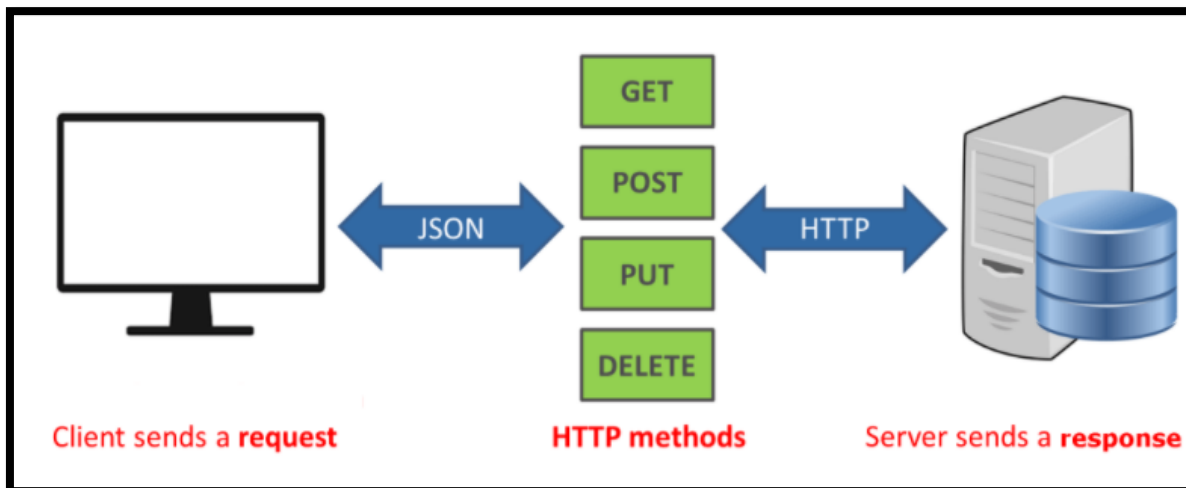
Ilustración 21 Arquitectura métodos de petición Http
