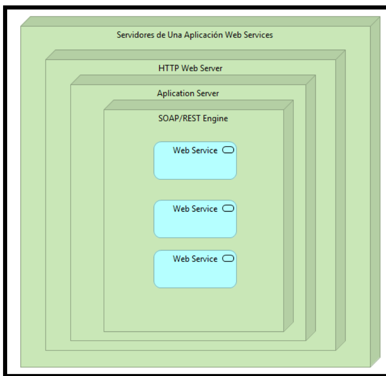
Ilustración 9 Roles, estructura de servidores en una aplicación Web Service
